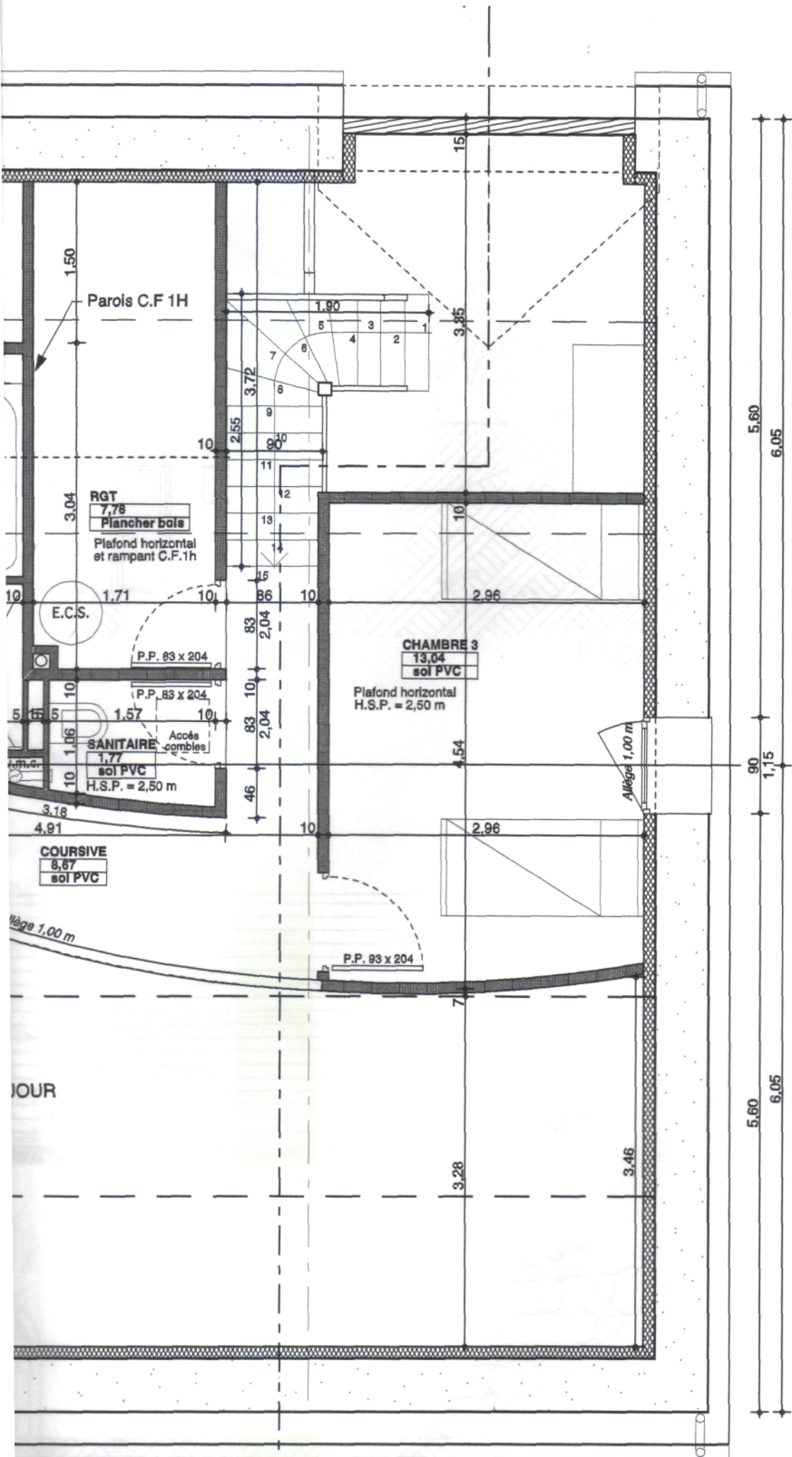
PLAN NIVEAU 2 - Ech 1/50°
