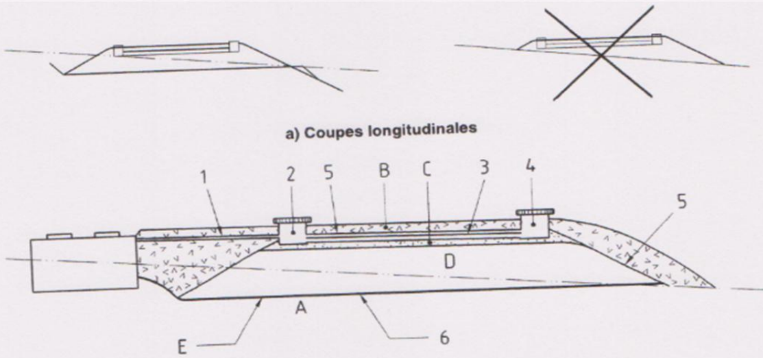
Figure 9 — Exemple de tertre d'infiltration hors sol
