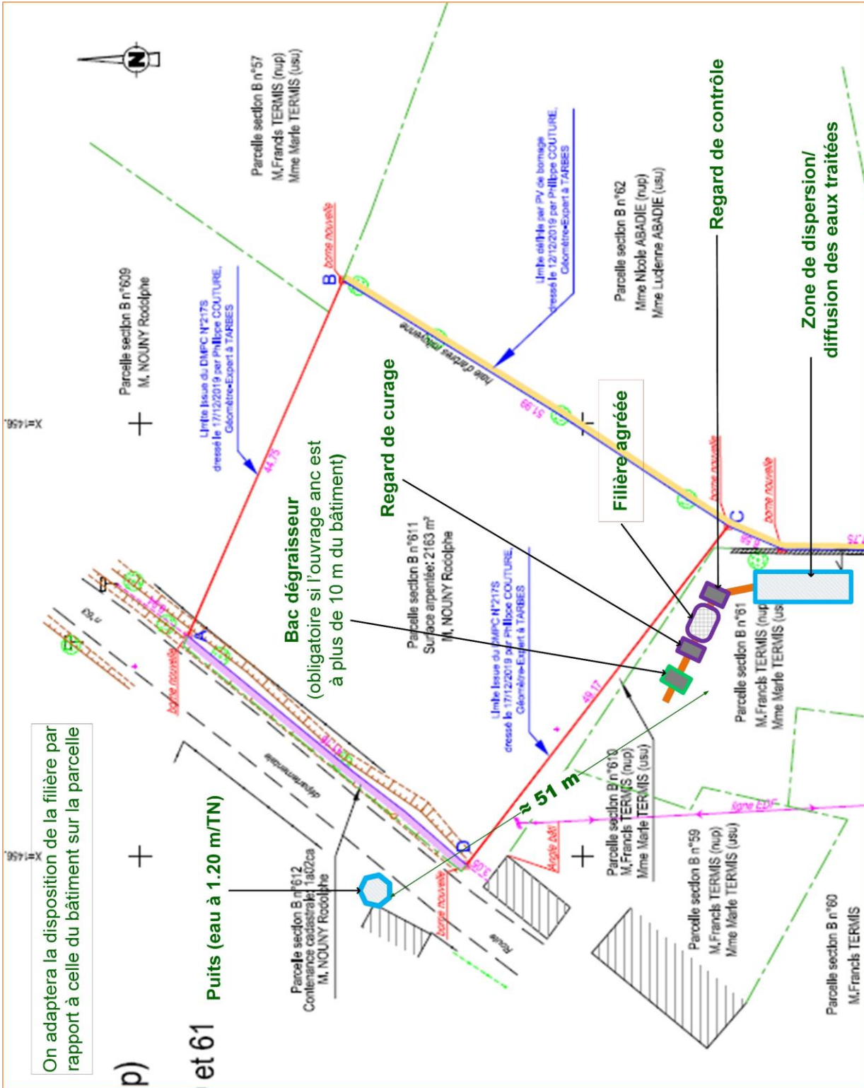
PLAN D'ASSAINISSEMENT : FILIERE AGREEE (FILTRE COMPACT OU SYSTEME COMPACT) AVEC REJET DANS LA ZONE DE DISPERSION/ DIFFUSION
