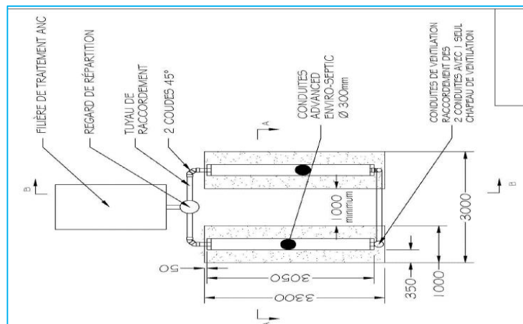
Schéma de principe du PITT
