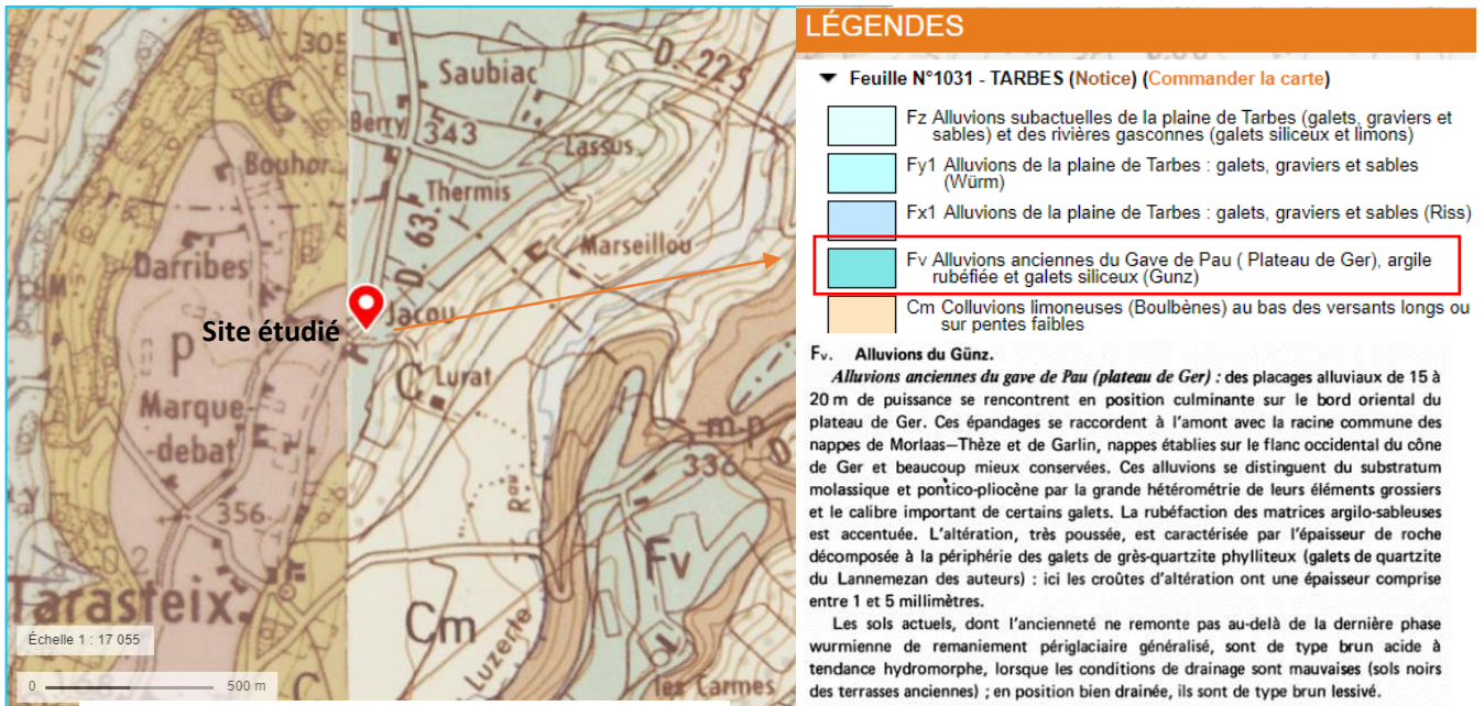
Extrait de carte géologique du secteur de l'étude
