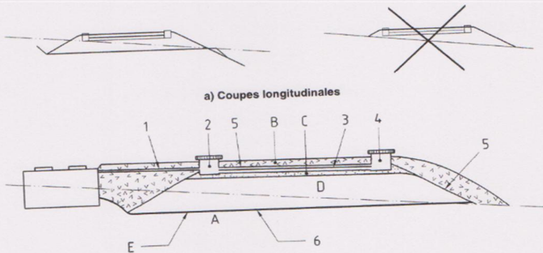
Figure 9 — Exemple de terte d'infiltration hors sol
