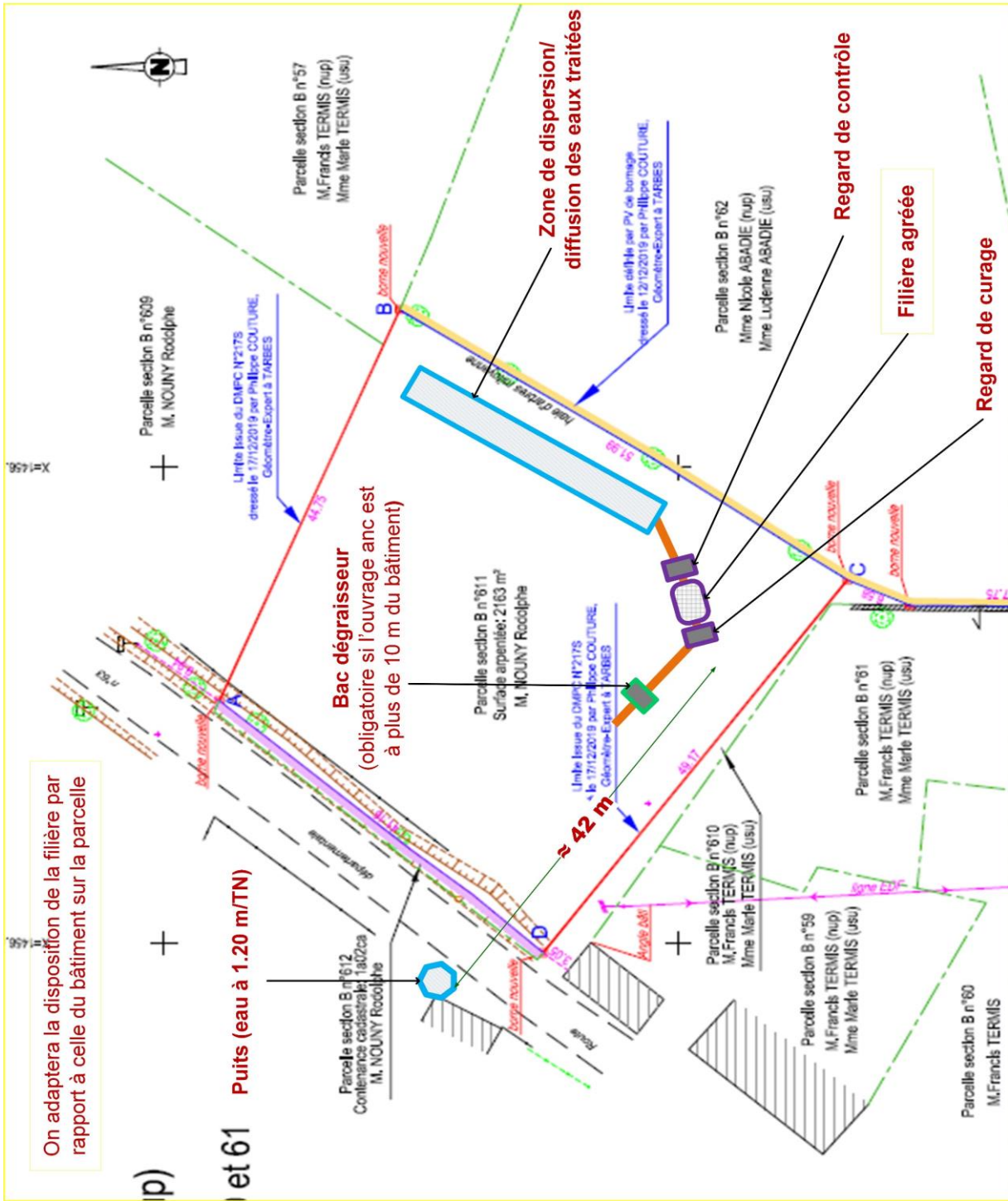
PLAN D'ASSAINISSEMENT : FILIERE AGREEE (FILTRE COMPACT OU SYSTÈME COMPACT) AVEC REJET DANS LA ZONE DE DSIPERSION/ DIFFUSION
