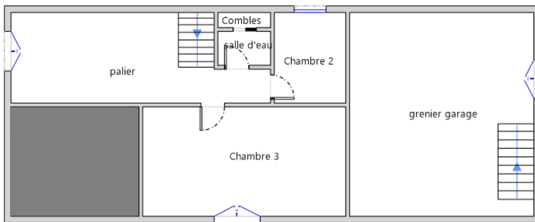
1er Etage
