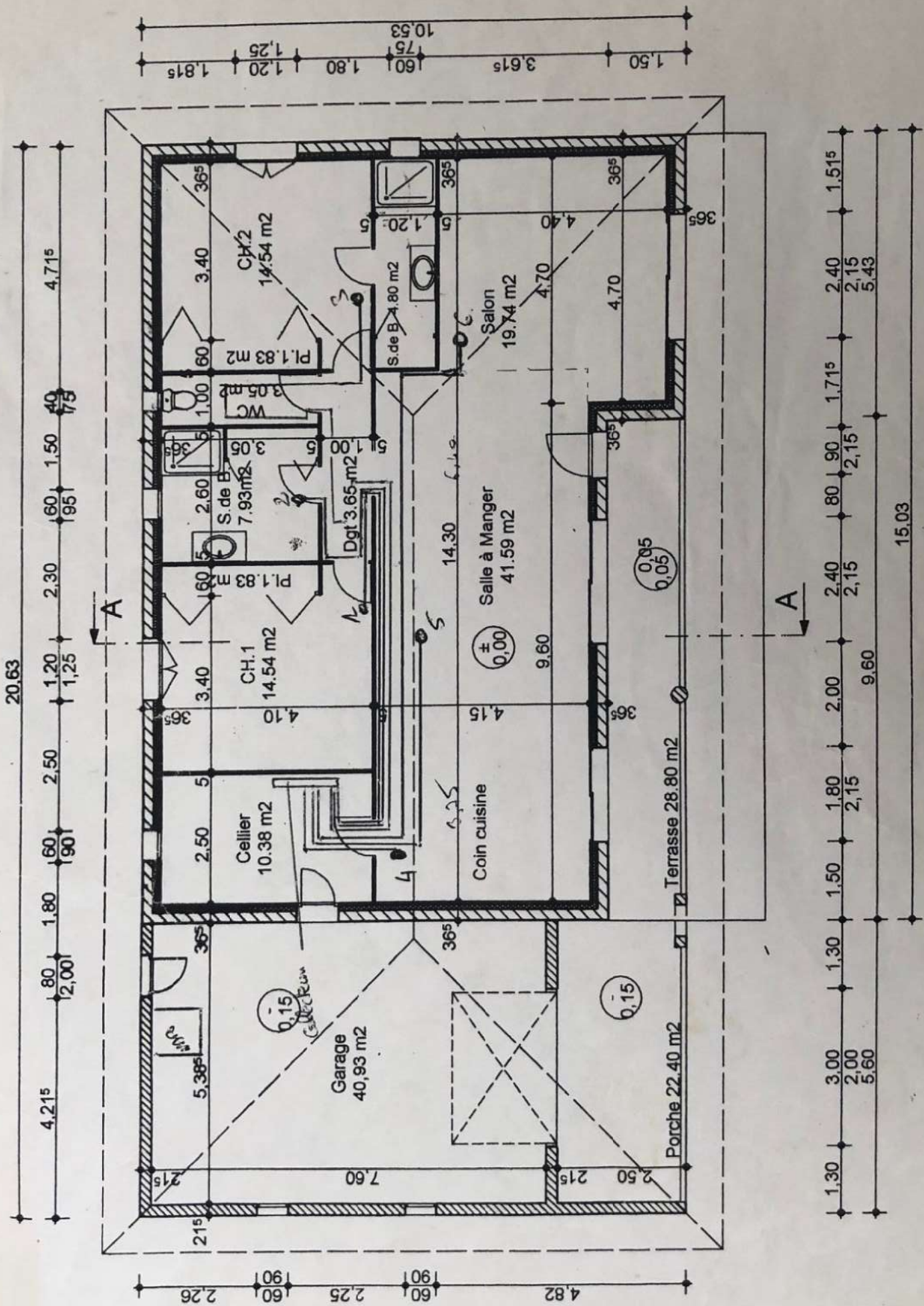
Vue en Plan Echelle : 1/100
