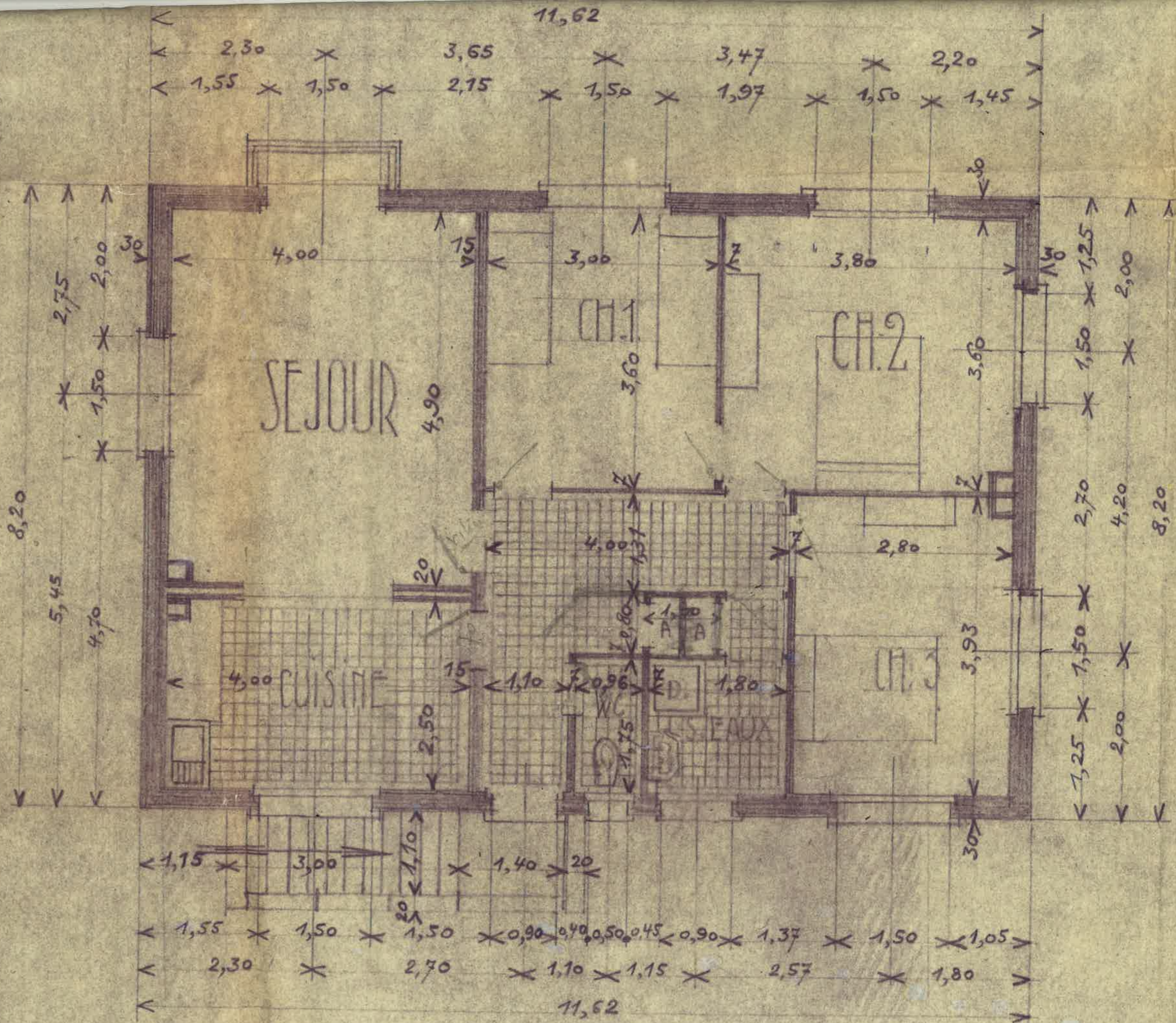
PLAN DU REZ-DE-CHAUSSEE.
