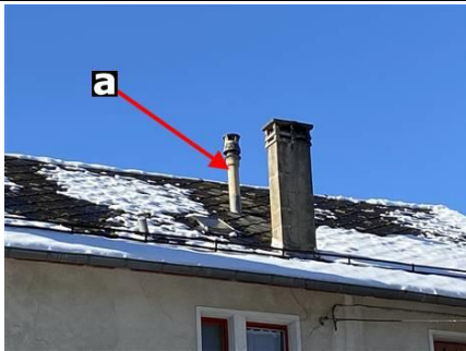
Photo n° PhA013 Localisation : Toiture - Couverture Ouvrage : Conduits en toiture et façade Partie d'ouvrage : Conduits de fumée en amiante-ciment Description : Conduits de fumée en amiante-ciment Localisation sur croquis : ZPSO-013
