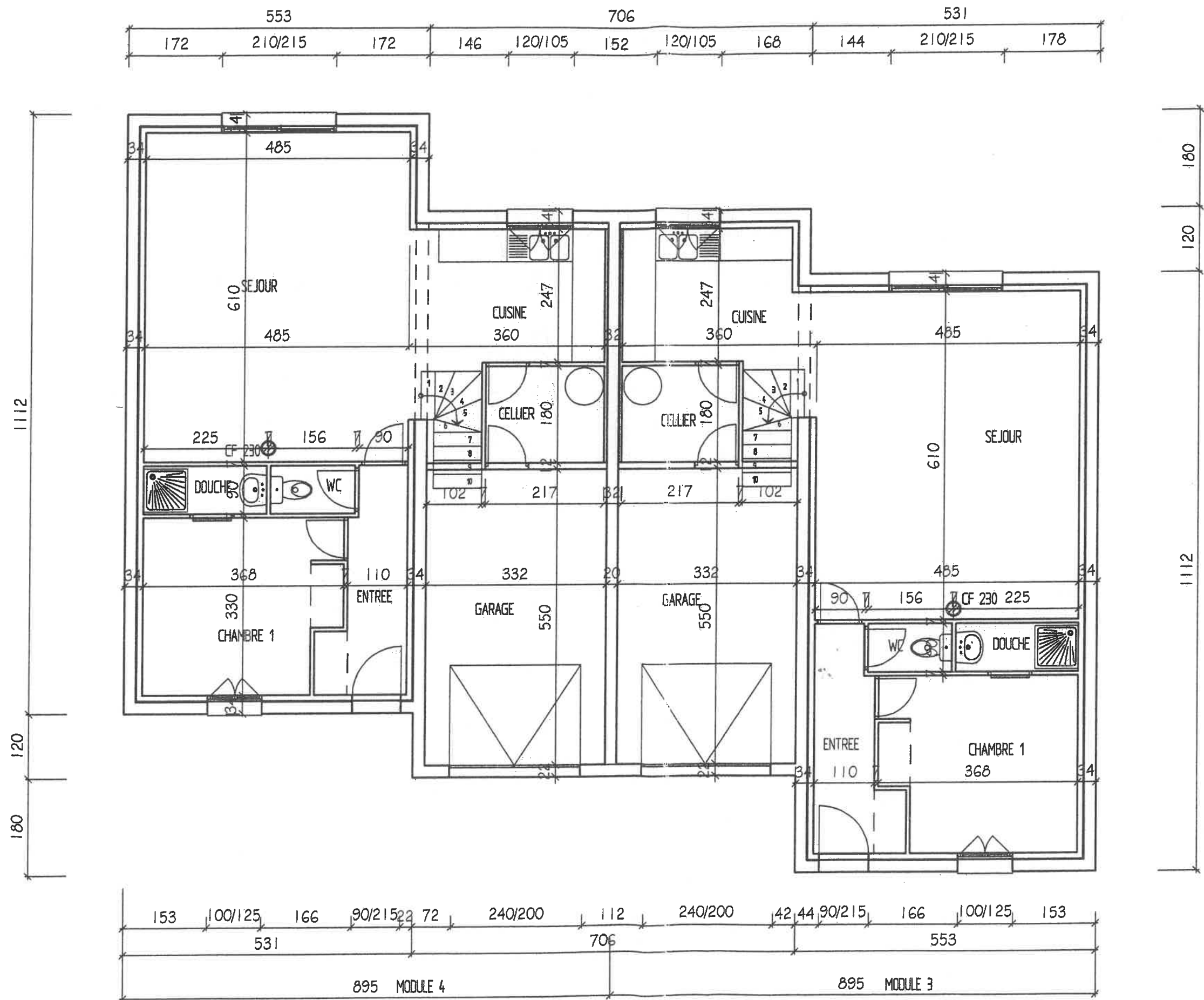
PLAN DU REZ-DE-CHAUSSEE Ech: 1/75e
