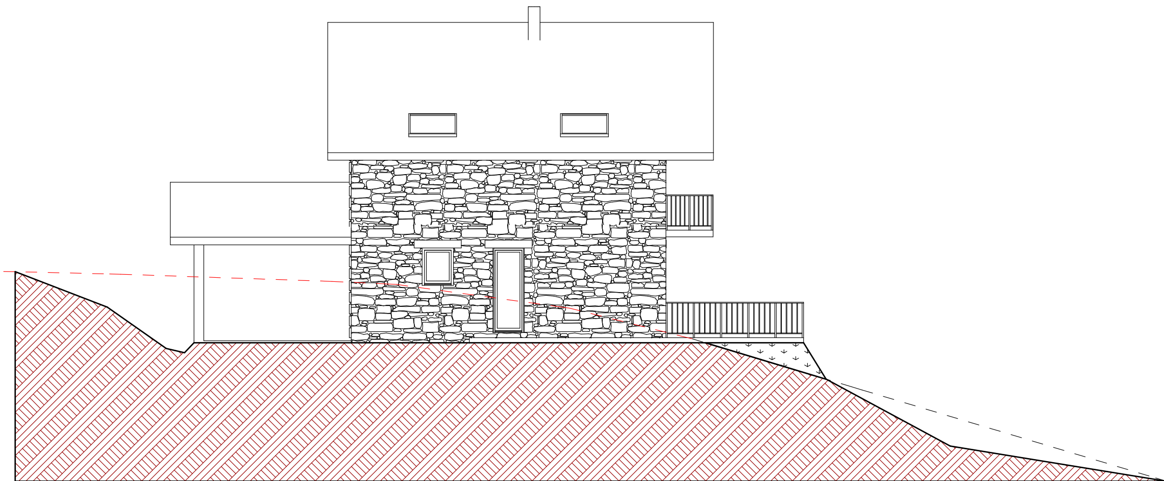
FACADE OUEST
