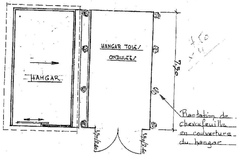
VUE EN PLAN (éch. 0.01 p.m.)
