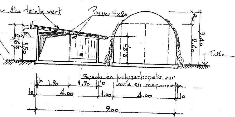
COUPE TRANSVERSALE (éch. 0.01 p.m.)
